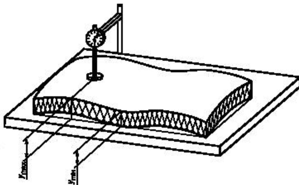
Рисунок 2 — Измерение максимального и минимального расстояний
