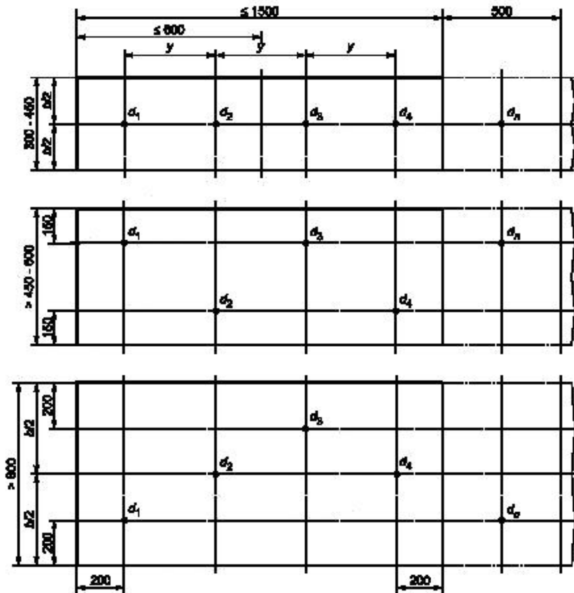
Рисунок 2 — Расположение точек, в которых проводят измерения
