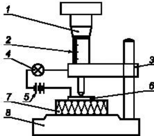
1 — винтовой микрометр; 2 — шкала с делениями в миллиметрах; 3 — регулируемая опора; 4 — лампа; 5 — батарея; 6 — алюминиевая пластина площадью 10 см 2 ; 7 — образец для измерения; 8 — основание
